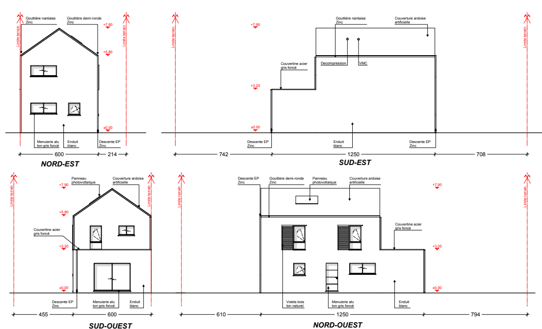
FACADES Echelle : 1/50
