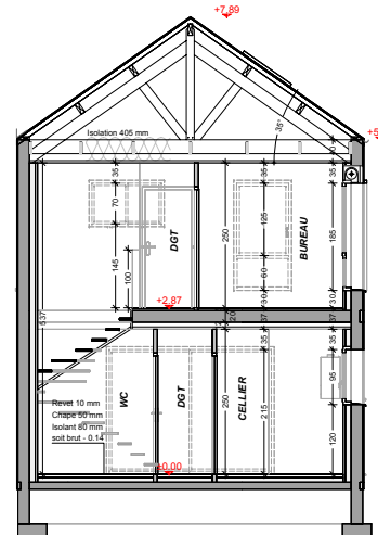
COUPE AA Echelle : 1/50
